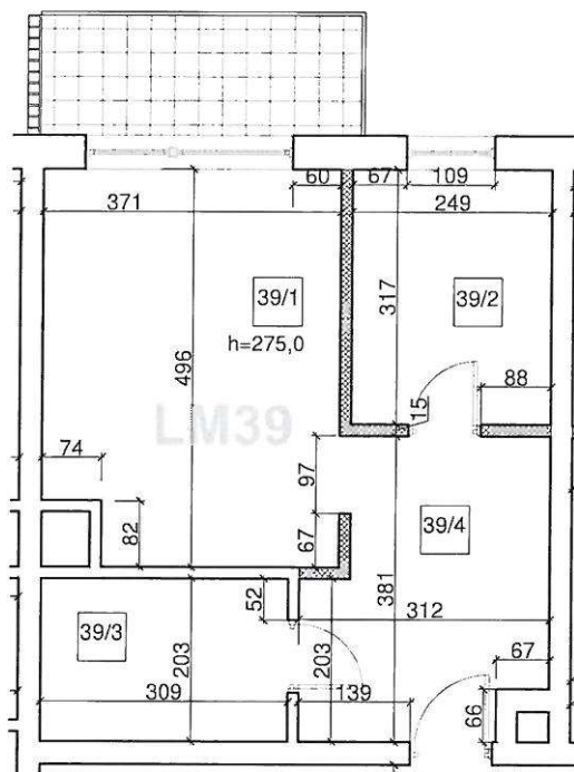
rzut piętra IV-budynek A skala 1:100
